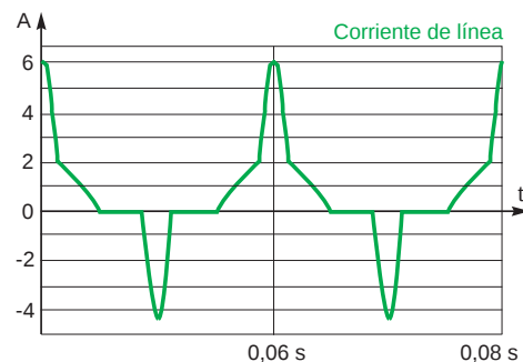
Fig. 2: Gráfica de la corriente absorbida.
