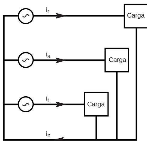
Fig. 12: Cargas monofásicas.
