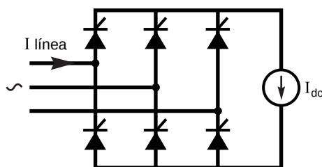
Fig. 36: Rectificador controlado que alimenta una carga que absorbe una corriente perfectamente plana.
