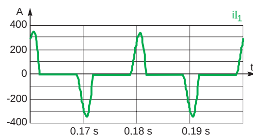
Fig. 27: Corriente de línea sin filtro.
