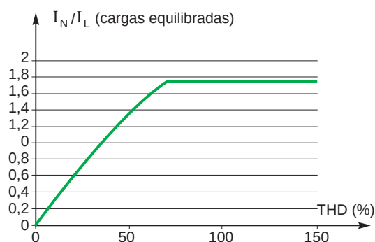
Fig. 19: Tasa de carga de la corriente de neutro (cargas equilibradas).
