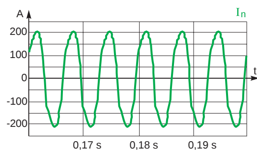
Fig. 18: Corriente en el neutro.
