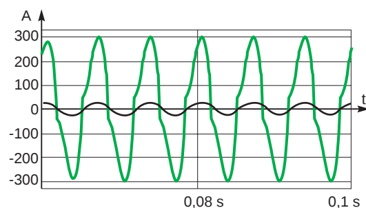
Fig. 25: Diferencia de amplitud de la corriente de neutro con y sin una reactancia en zigzag.
