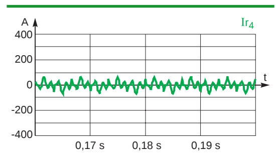
Fig. 31: Corriente de neutro con filtro.
