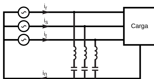
Fig. 33: Filtro pasivo de 3 er orden.
