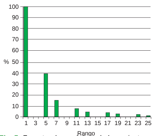
Fig. 7: Espectro de armónicos de la corriente absorbida en el ejemplo de la figura 5.
