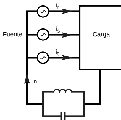
Fig. 26: Filtro de 3 er orden en el neutro.
