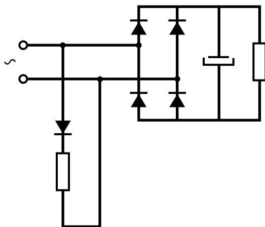
Fig. 1: Ejemplo de una carga cualquiera no lineal (no simétrica).
