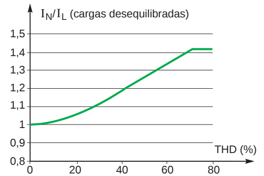
Fig. 21: Tasa de carga de la corriente de neutro (cargas desequilibradas).
