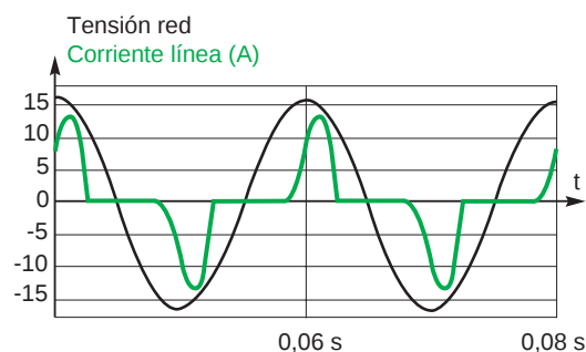
Fig. 9: Gráfica de la corriente absorbida en el esquema de la figura 8.
