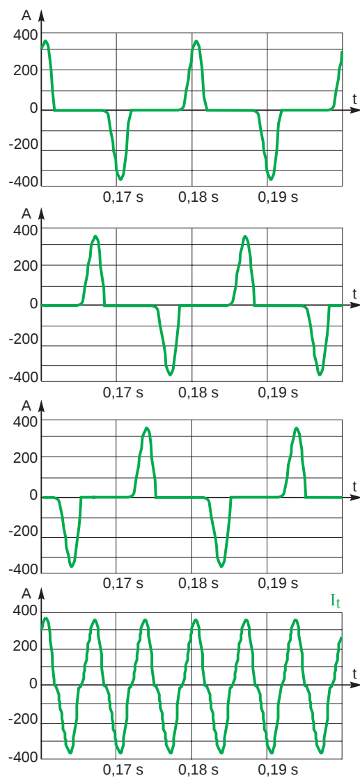
Fig. 14: Corrientes de las fases y de neutro que alimentan cargas monofásicas no lineales.
