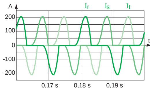
Fig. 17: Corrientes de las 3 fases.
