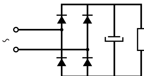
Fig. 8: Rectificador monofásico con filtro capacitativo.
