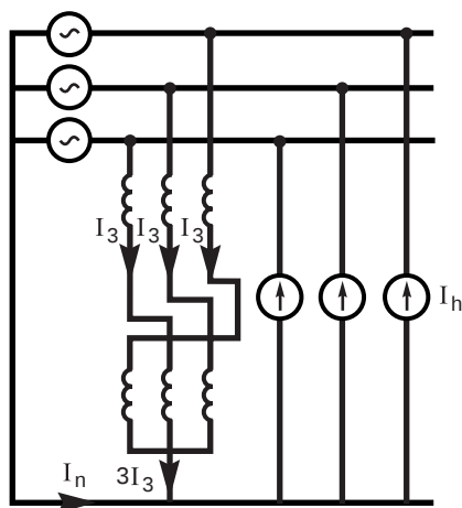
Fig. 24: Reactancia zigzag.
