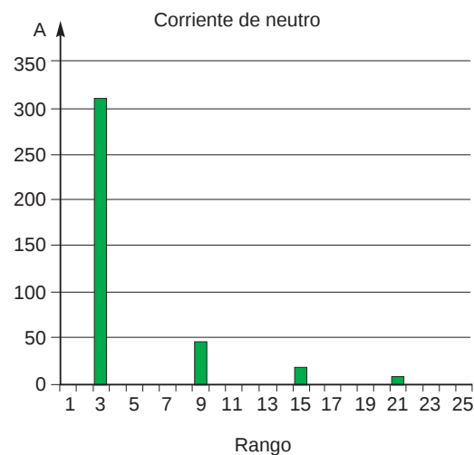
Fig. 16: Espectro de la corriente de neutro absorbida por cargas monofásicas no lineales.
