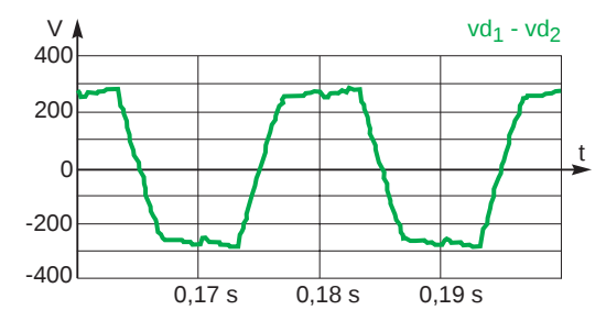
Fig. 32: Tensión simple con filtro.
