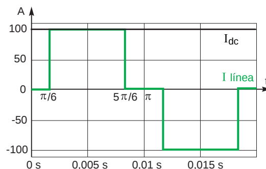
Fig. 37: Corriente de alimentación.
