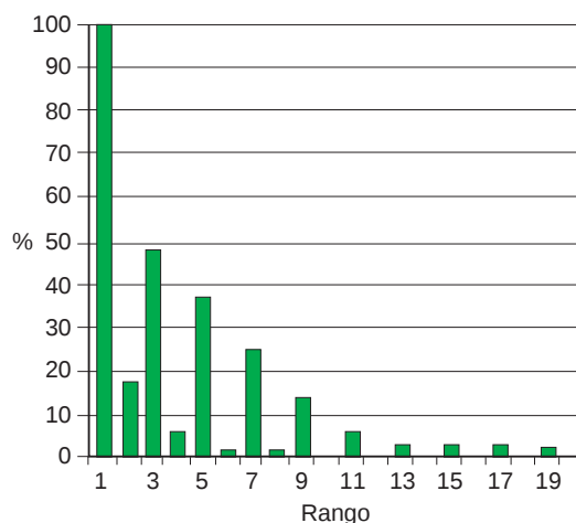
Fig. 3: Espectro de la corriente absorbida.
