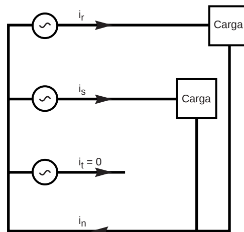
Fig. 20: Cargas desequilibradas.
