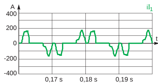
Fig. 30: Corriente de línea con filtro.
