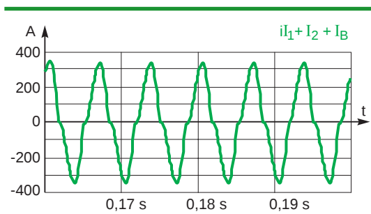
Fig. 28: Corriente de neutro sin filtro.
