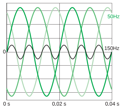
Fig. 13: Corrientes trifásicas a 50 Hz y 150 Hz absorbidas por cargas lineales.
