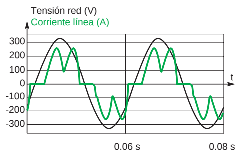
Fig. 6: Gráfica de la corriente absorbida en el esquema de la figura 5.
