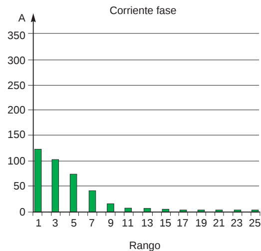
Fig. 15: Espectro de la corriente de fase que alimenta cargas monofásicas no lineales.
