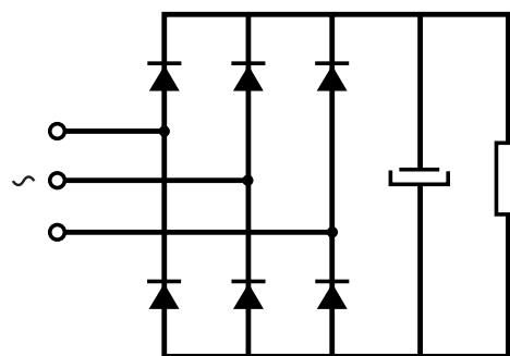
Fig. 5: Puente rectificador trifásico con filtro capacitativo.
