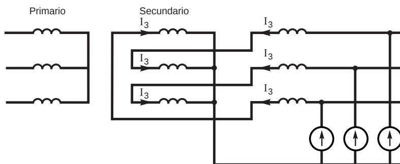
Fig. 23: Corrientes armónicas de 3 er orden en un transformador con el secundario en zigzag.
