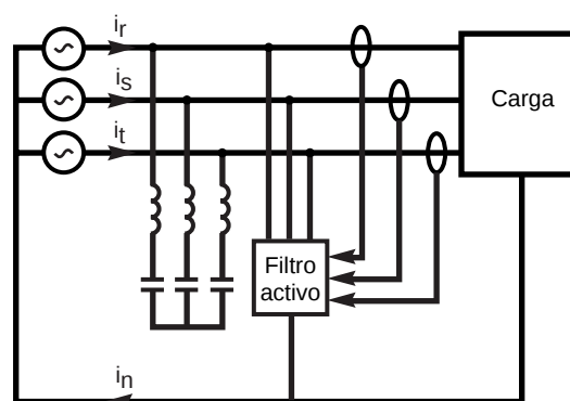
Fig. 35: Filtro híbrido.
