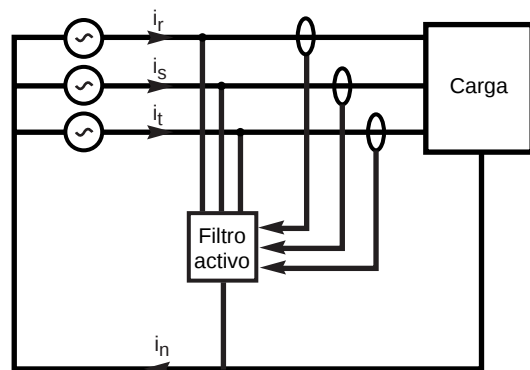
Fig. 34: Filtro activo.
