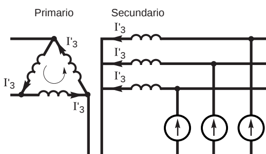
Fig. 22: Corrientes armónicas de 3 er orden en un transformador triángulo-estrella.
