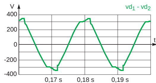
Fig. 29: Tensión simple sin filtro.
