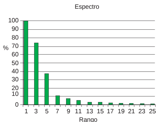
Fig. 10: Espectro de armónicos de la corriente absorbida en el esquema de la figura 8.
